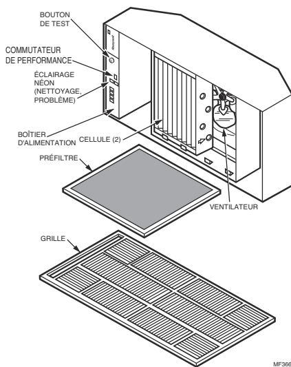
Fig. 4. Emplacement du boîtier d'alimentation sur les Épurateurs d'air F57. Ouvrir pour accéder l'alimentation.
