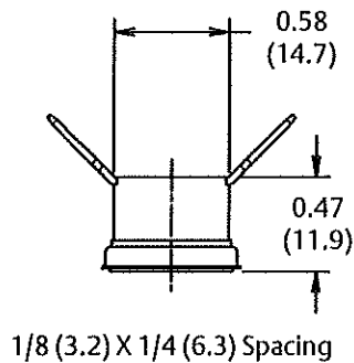
TX, TXE, TXH Surface Mount
