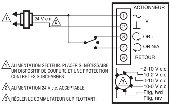
Fig. 15. MS7505 pour action flottante (réglage en mode flottant)
