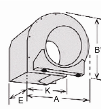
Downblast (DB)*
