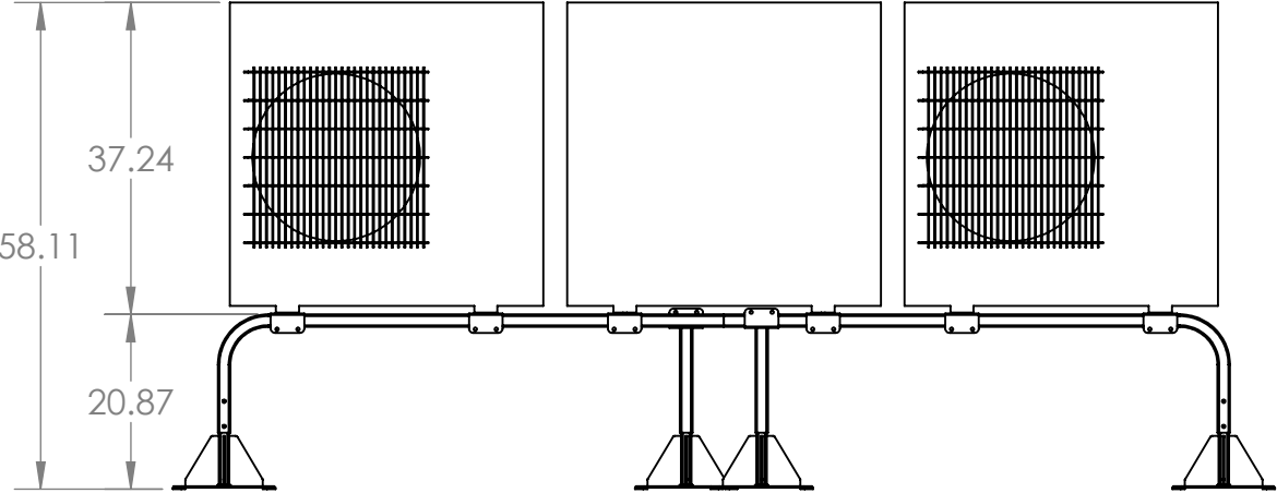
THREE (3) MINI SPLIT CONFIGURATION
